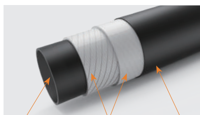
内衬层 Inside layer 缠绕增强层 (丝类) Winding reinforcement layer(fiber type) 保护层 Protective layer
